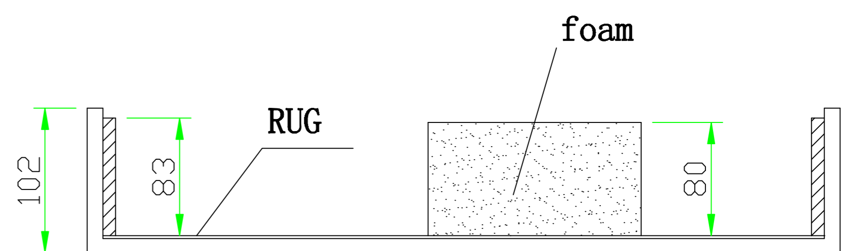
B—B
